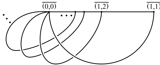
Fig. 2. Hawaiian ropes HR.
